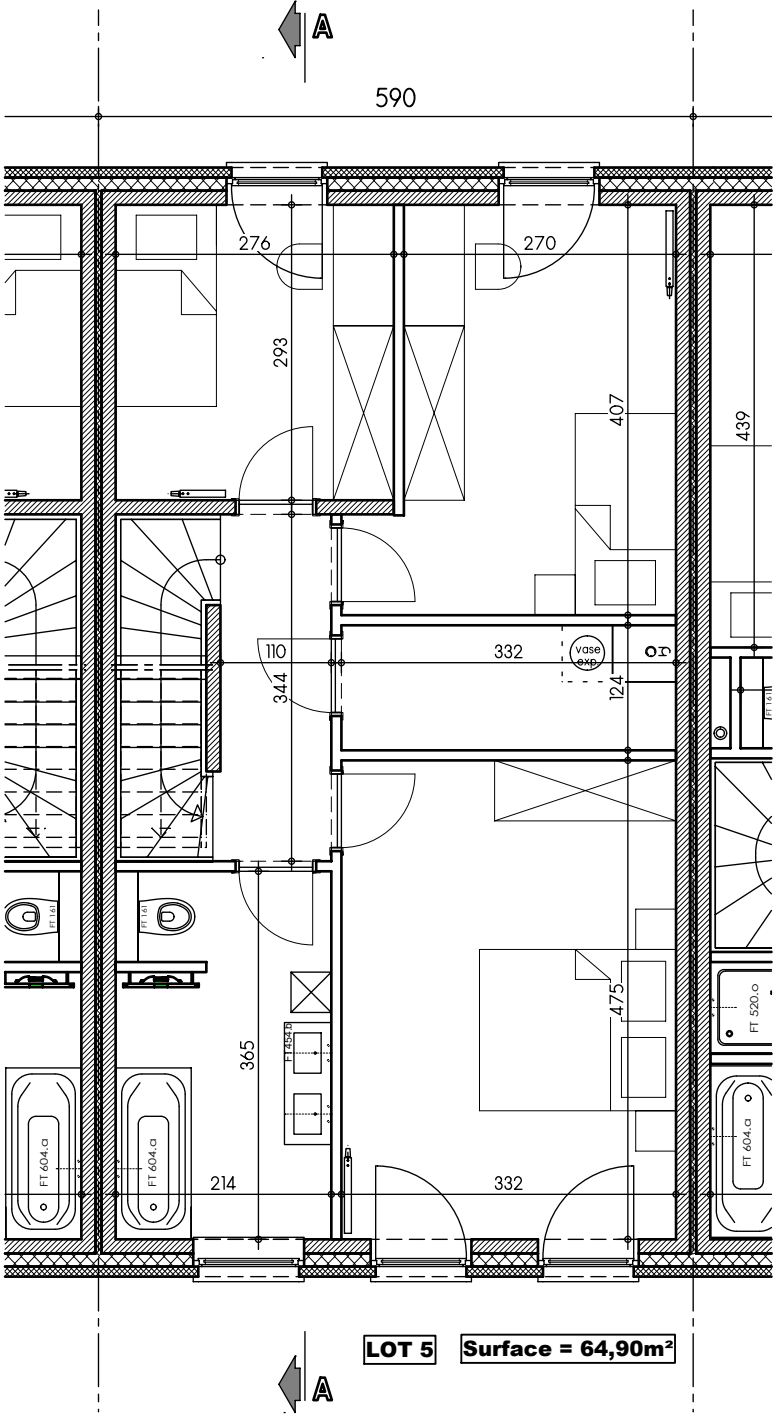
PLAN ETAGE
