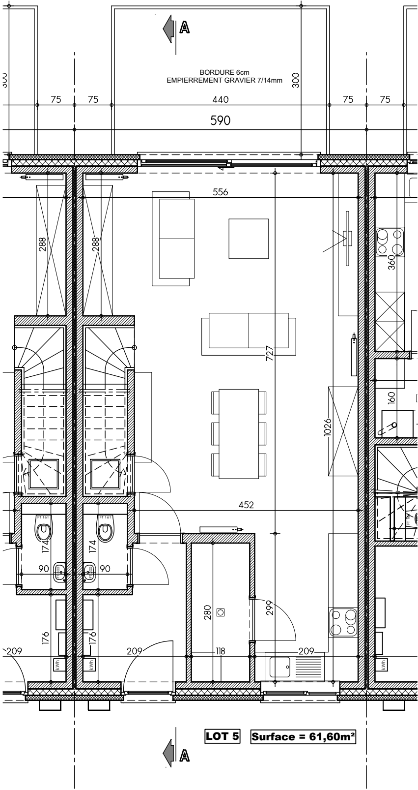
PLAN REZ-DE-CHAUSSEE
